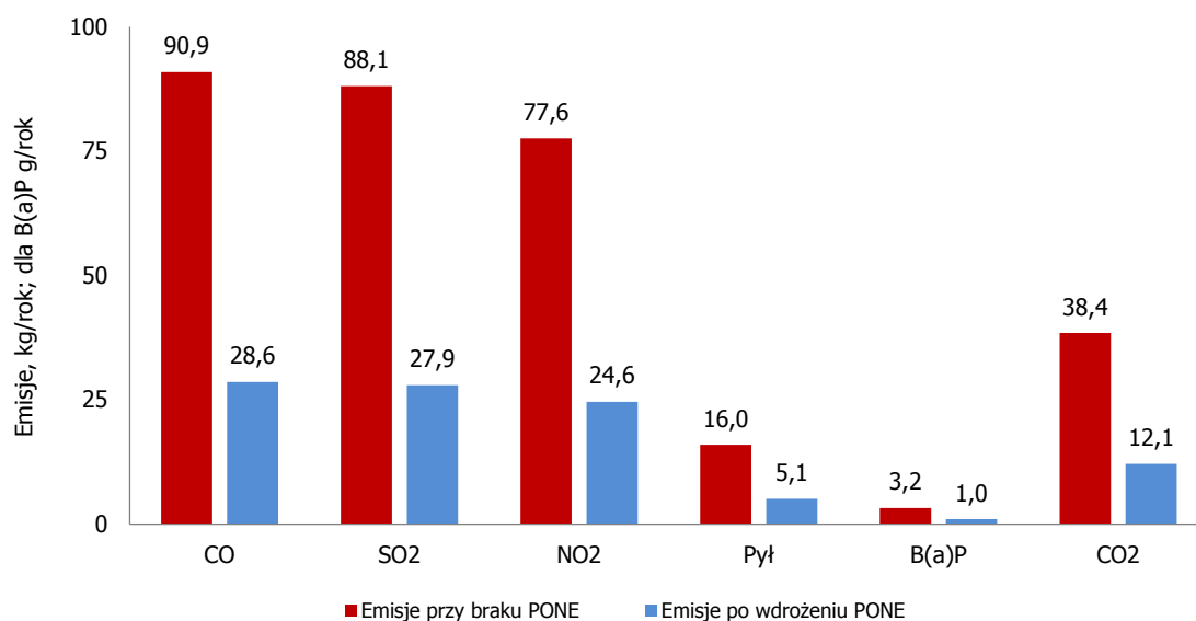
Rysunek 4.4 Roczne emisje substancji szkodliwych do atmosfery w budynkach objętych programem w 2014 roku, w których dokonano montażu kolektorów słonecznych oraz pomp ciepła na potrzeby c.w.u. (przed realizacją i po montażu)
