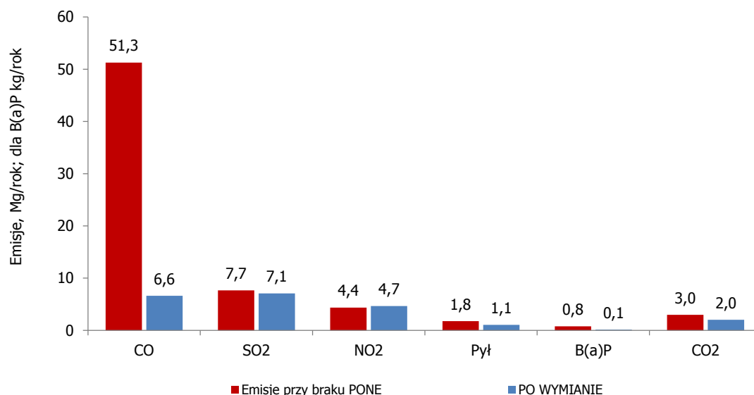
Rysunek 4.2 Roczne emisje substancji szkodliwych do atmosfery w budynkach istniejących objętych programem w 2014 roku (przed realizacją i po wymianie)
