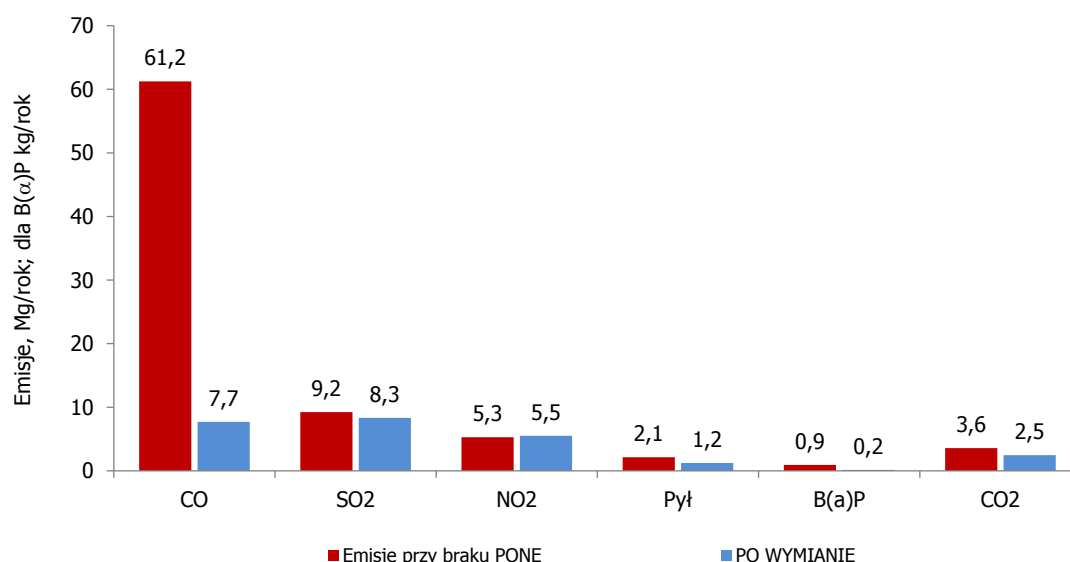
Rysunek 4.5 Roczne emisje substancji szkodliwych do atmosfery w budynkach objętych programem ograniczenia niskiej emisji w 2014 roku (przed realizacją i po realizacji)
