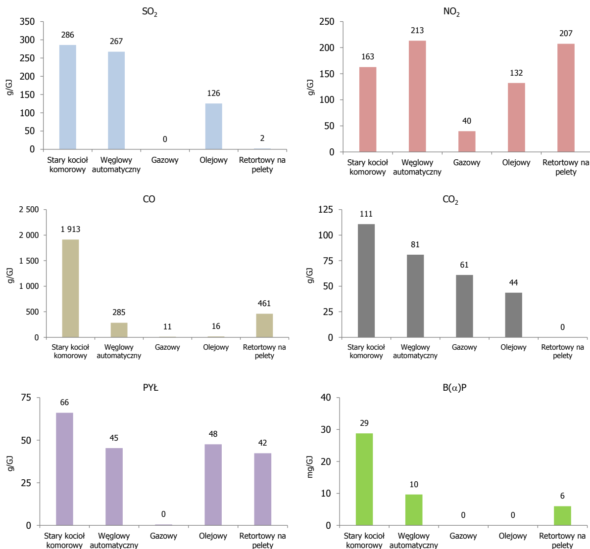
Rysunek 4.1 Emisja jednostkowa z poszczególnych źródeł ciepła
