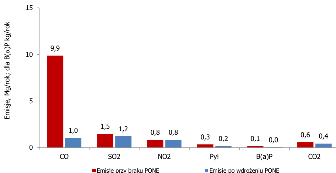
Rysunek 4.3 Roczne emisje substancji szkodliwych do atmosfery w budynkach nowobudowanych objętych programem w 2014 roku (przed realizacją i po montażu)
